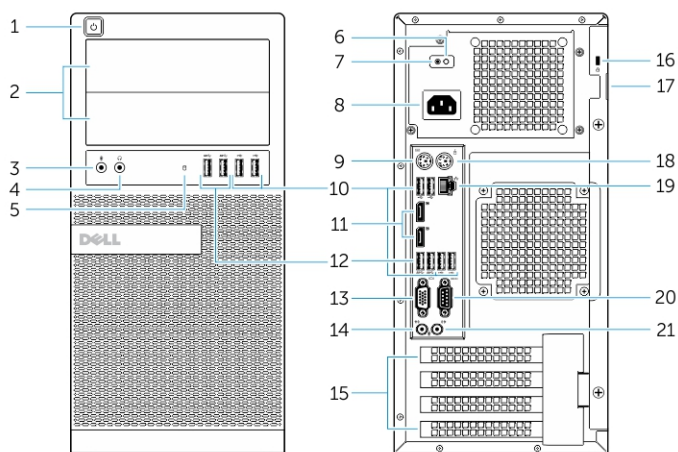
Figur 1. Minitårn sett forfra og bakfra
